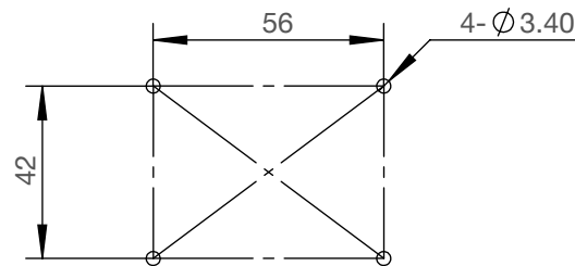
安装尺寸
